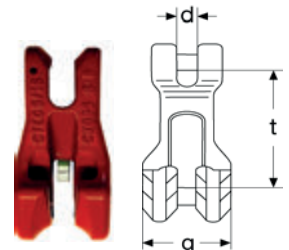
Verkürzungsklaue mit Sicherung
