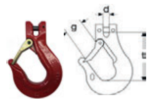
Gabelkopfhaken
